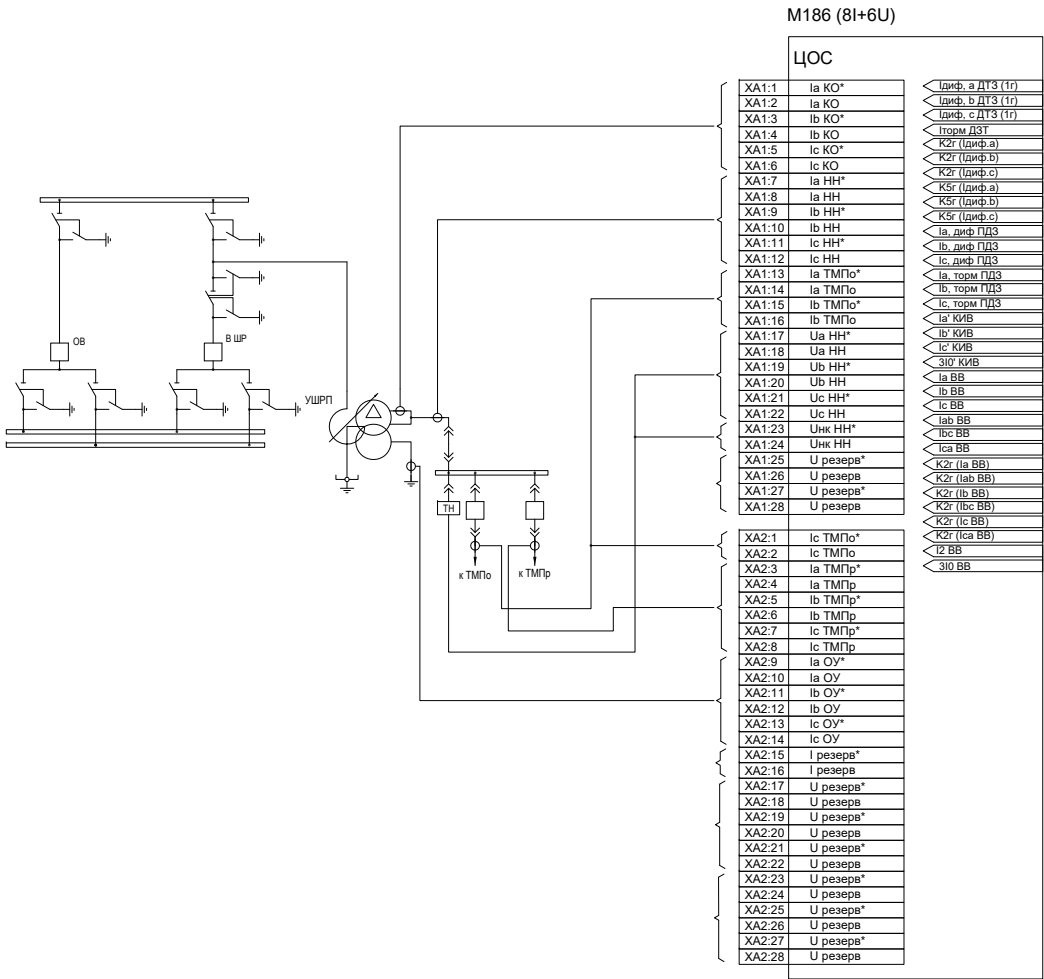
Рисунок Б.1 – Вариант подключения аналоговых цепей ТТ и ТН к устройству
