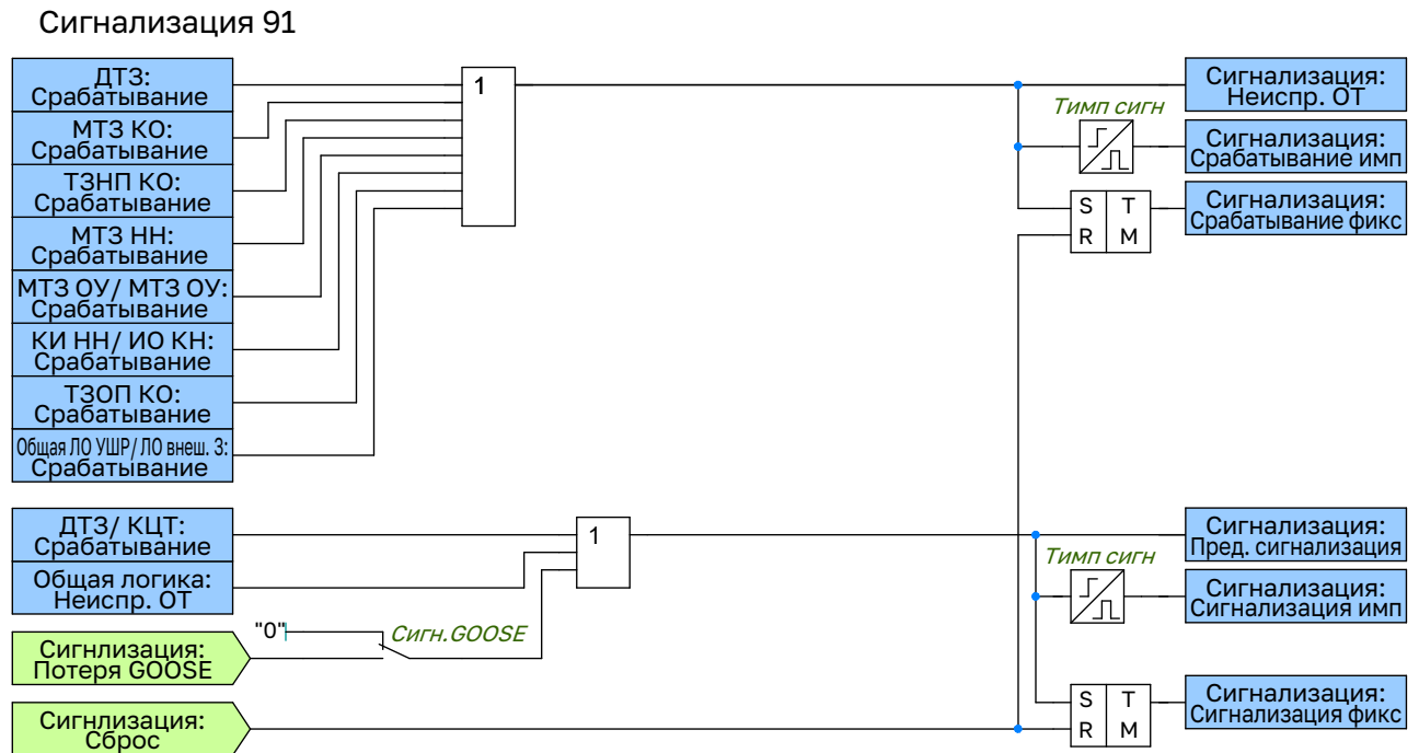
Рисунок 2.18 – Функциональная схема логики сигнализации
