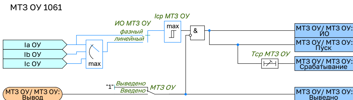
Рисунок 2.12 – Функциональная схема логики МТЗ ОУ
